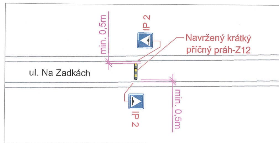
DETAIL UMÍSTĚNÍ PŘÍČNÉHO PRAHU
