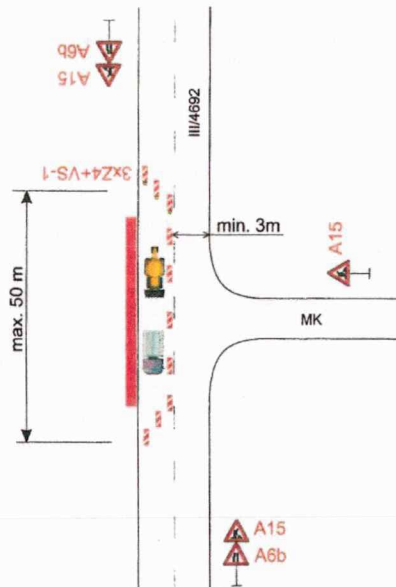
Stavba chodníku a zálivu pro BUS
