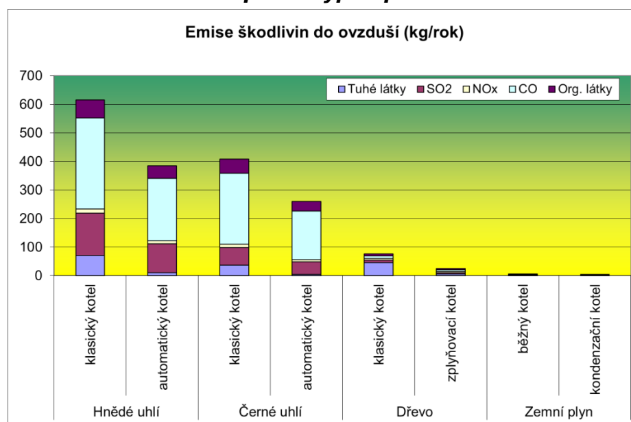
Graf Téma aglomerace: Životní prostředí (kvalita ovzduší).21: Emise škodlivin do ovzduší podle typů spalování
