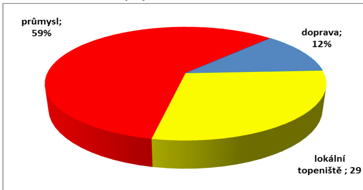
Graf Téma aglomerace: Životní prostředí (kvalita ovzduší).20: Odhad podílu zdrojů na emisní zátěž částicemi PM10 v ORP Ostrava při teplotě -7°C, transformace dle výšky komína
