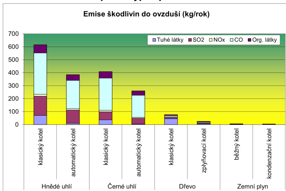
Graf Téma aglomerace: Životní prostředí (kvalita ovzduší).24: Emise škodlivin do ovzduší podle typů spalování
