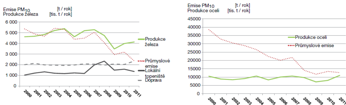
Graf Téma aglomerace: Životní prostředí (kvalita ovzduší).22: Vývoj emisí a výroby železa a oceli
